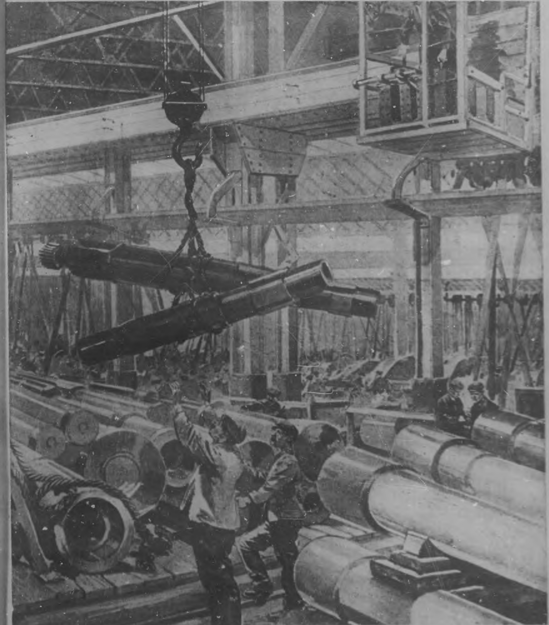
El interior de una gran fábrica inglesa y donde puede apreciarse la intensificación en la fabricación de pertrechos de guerra.
